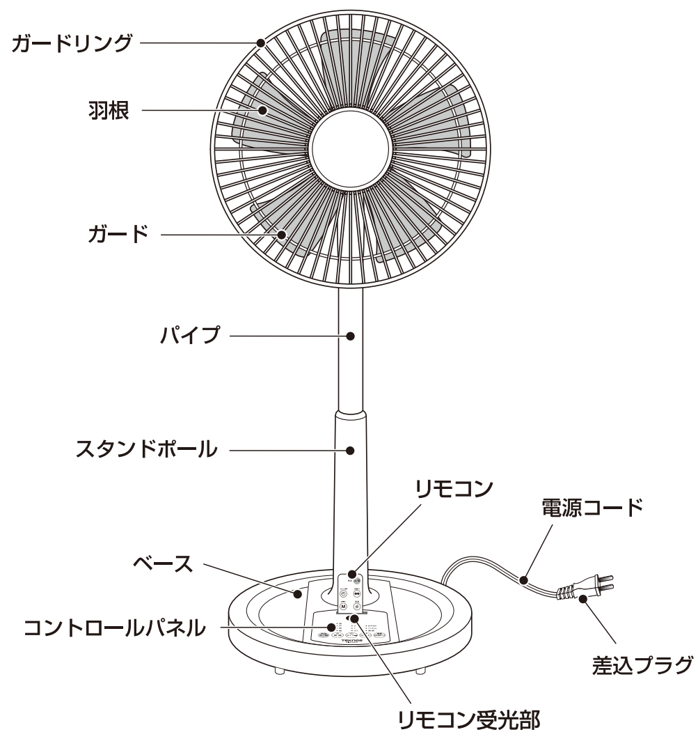
本体（正面）
